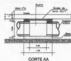
DETALHAMENTO DAS BOCAS DE LOBO
