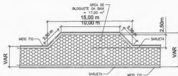
DETALHE TÍPICO DAS BAIS SEM ESCALA - UNIDADE m
