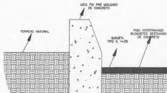
DETALHE ASSENTAMENTO MEIO FIO
