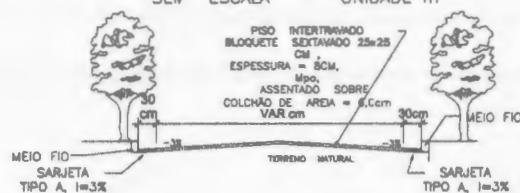
CORTE TÍPICO DA PISTA SEM ESCALA - UNIDADE m
