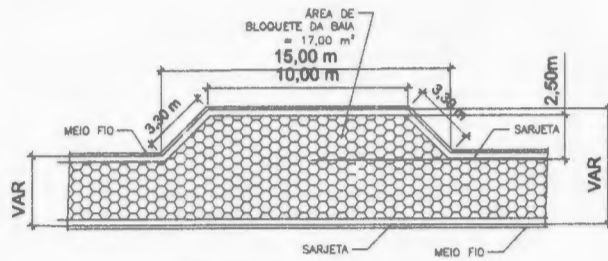
DETALHE TÍPICO DAS BAIAS SEM ESCALA - UNIDADE m
