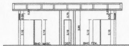
CORTE AA 1 : 100
