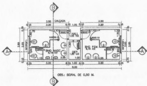
PLANTA BAIXA 1 : 100
